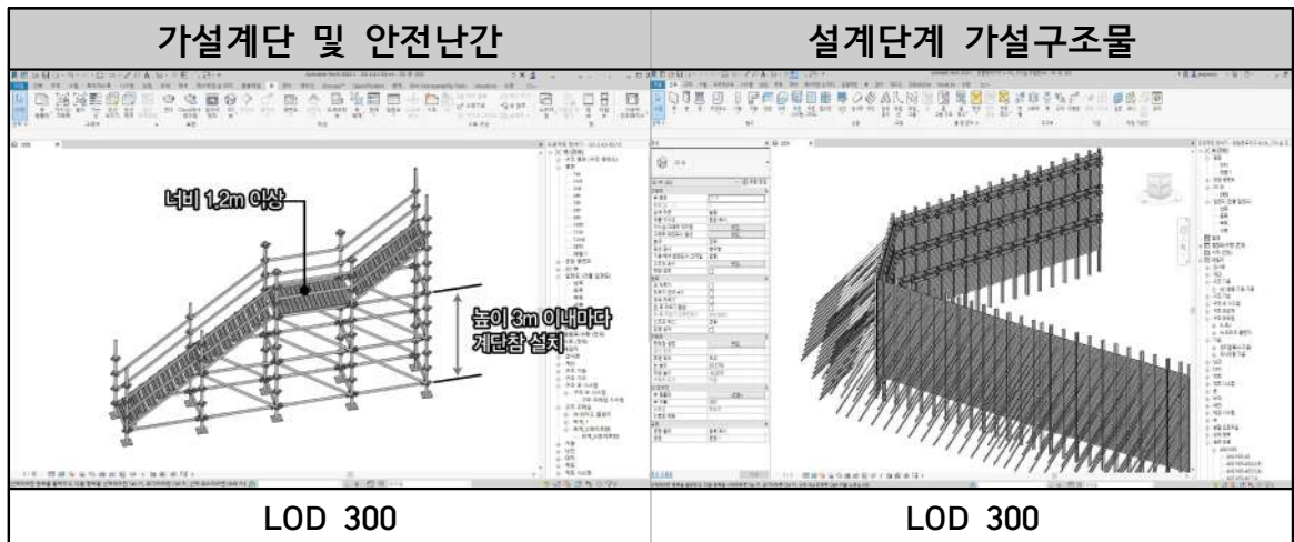
< 그림-19 > 가설구조물 BIM 모델 작성 예
