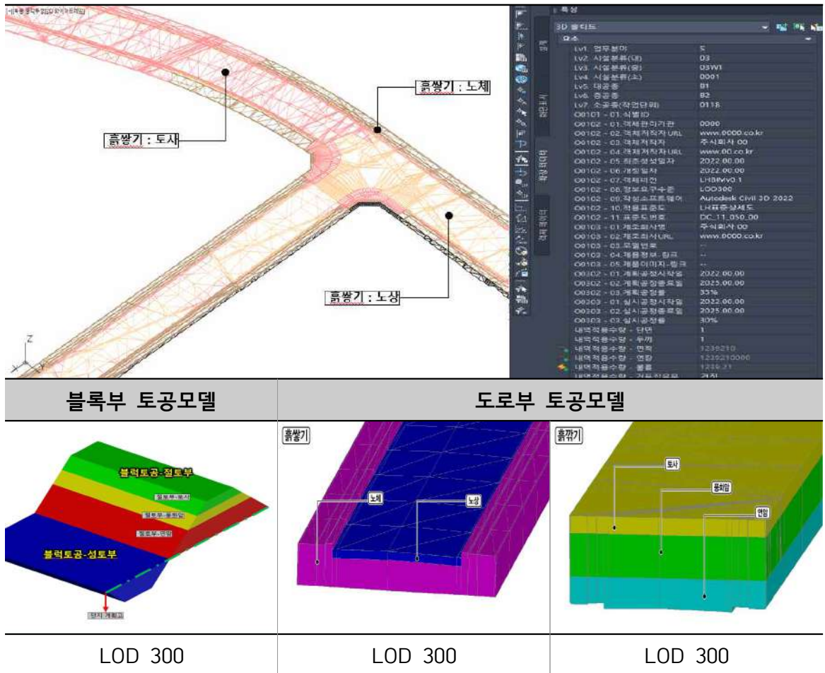
<그림-9> 토공시설 BIM 모델 작성 예
