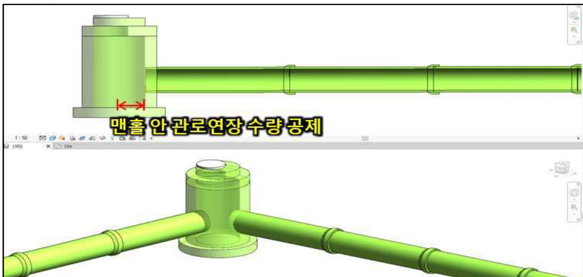
< 그림-13 > 관로시설 BIM 모델 배치 예
