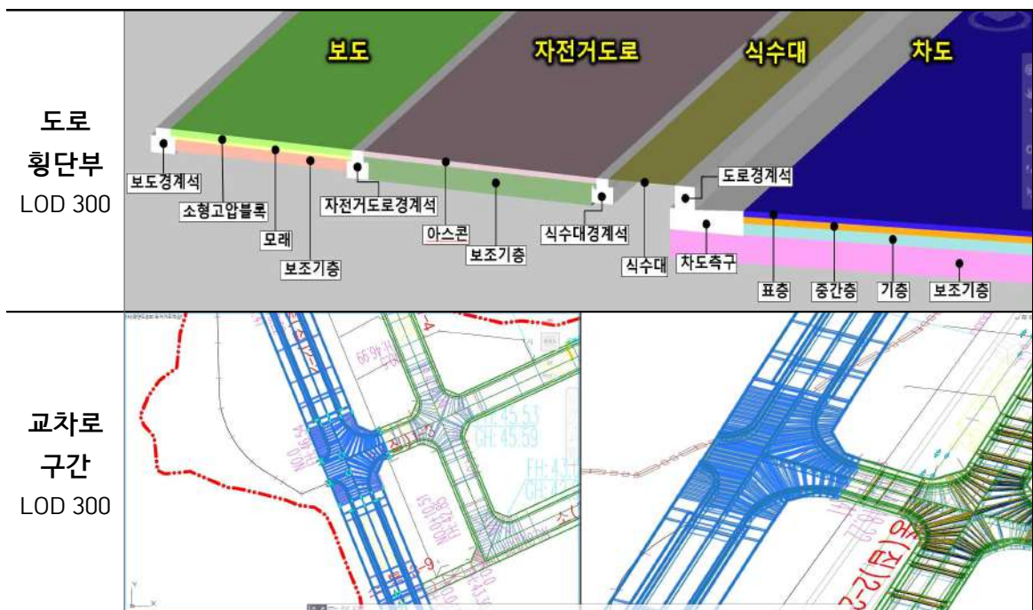
<그림-11> 도로시설 BIM 모델 작성 예
