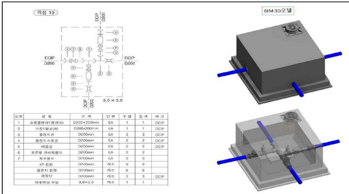
< 그림-14 > 상수시설 격점 상세도 BIM 모델 작성 예
