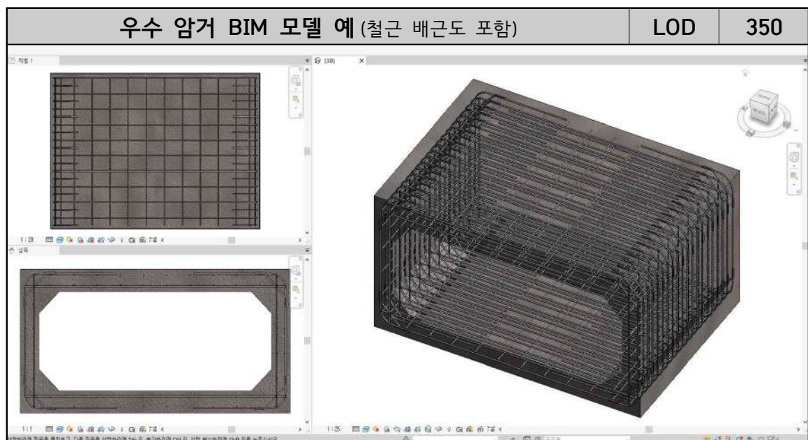
&lt;그림-16&gt; 구조물(암거, 철근 배근도 포함) BIM 모델 작성 예
