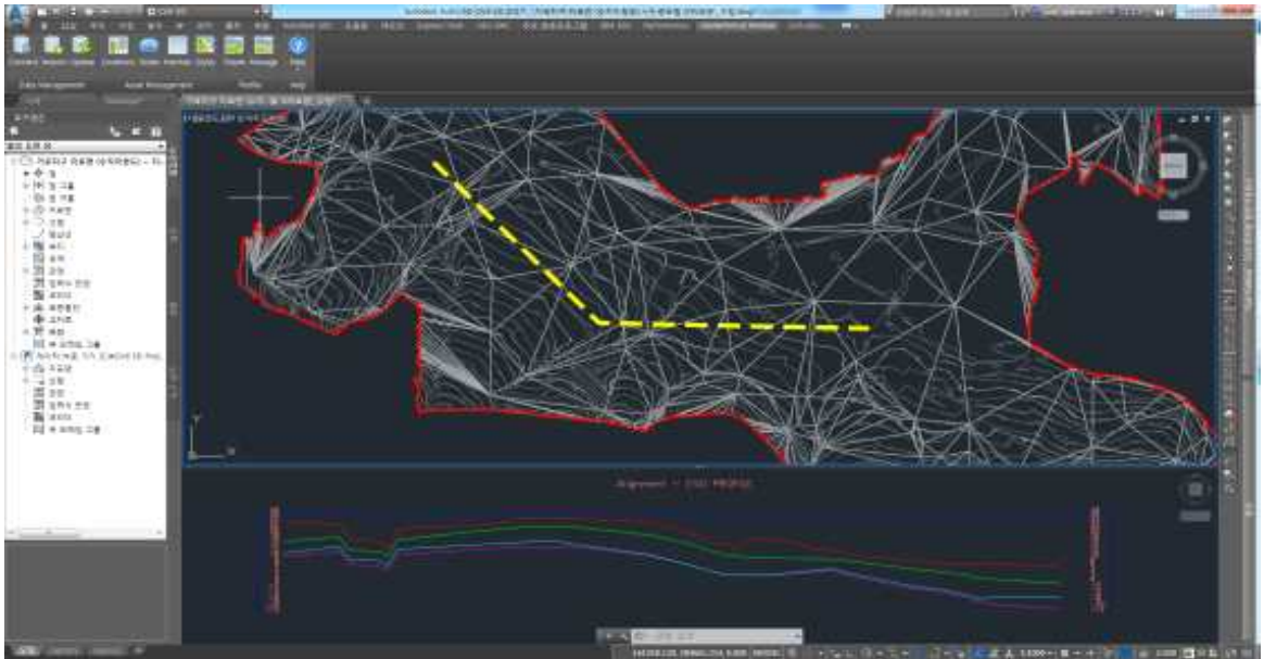
<그림-7> 3차원 지층 BIM 모델 구성 예
