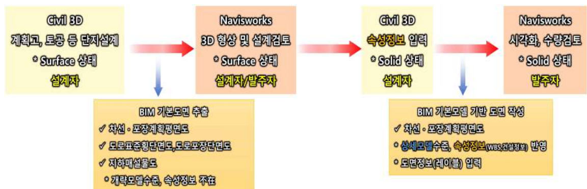
<그림-10> 도로시설 BIM 모델 구축 업무수행 흐름도
