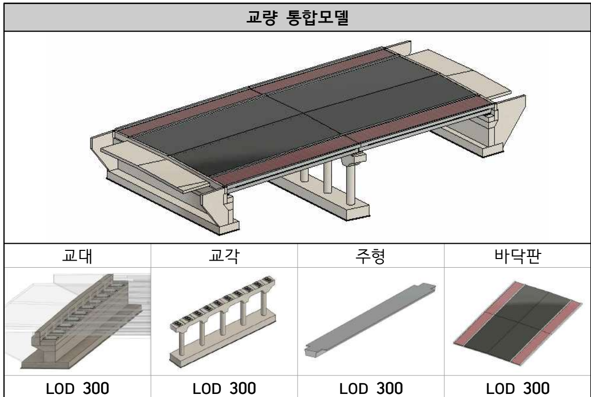
&lt; 그림-17 &gt; 구조물(교량) BIM 모델 작성 예
